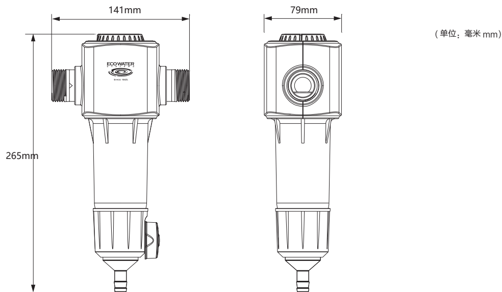
怡口牌 ESF102-M 型前置过滤器
